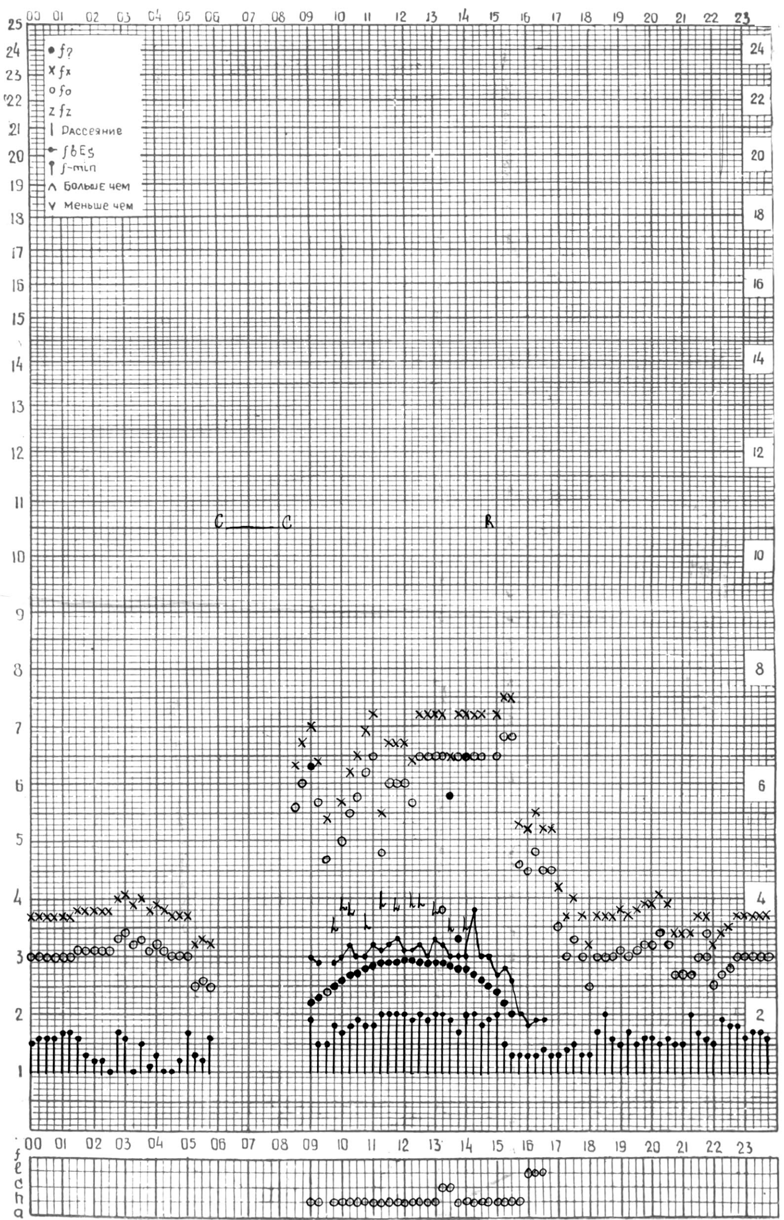
СТАНЦИЯ ТБИЛИСИ F-ГРАФИК ИОНОСФЕРНЫХ ДАННЫХ, ДАТА 16 ДЕКАБРЯ 1973г
