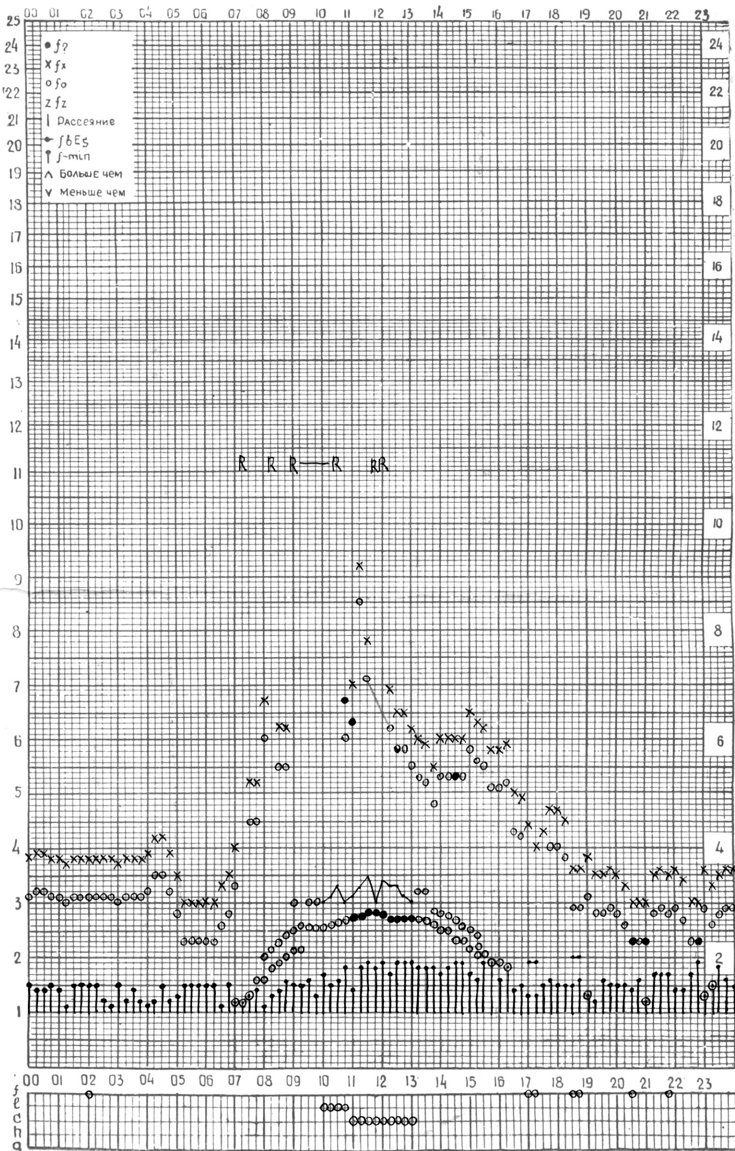
СТАНЦИЯ ТБИЛИСИ F-ГРАФИК ИОНОСФЕРНЫХ ДАННЫХ, ДАТА 15 ДЕКАБРЯ 1973 г
