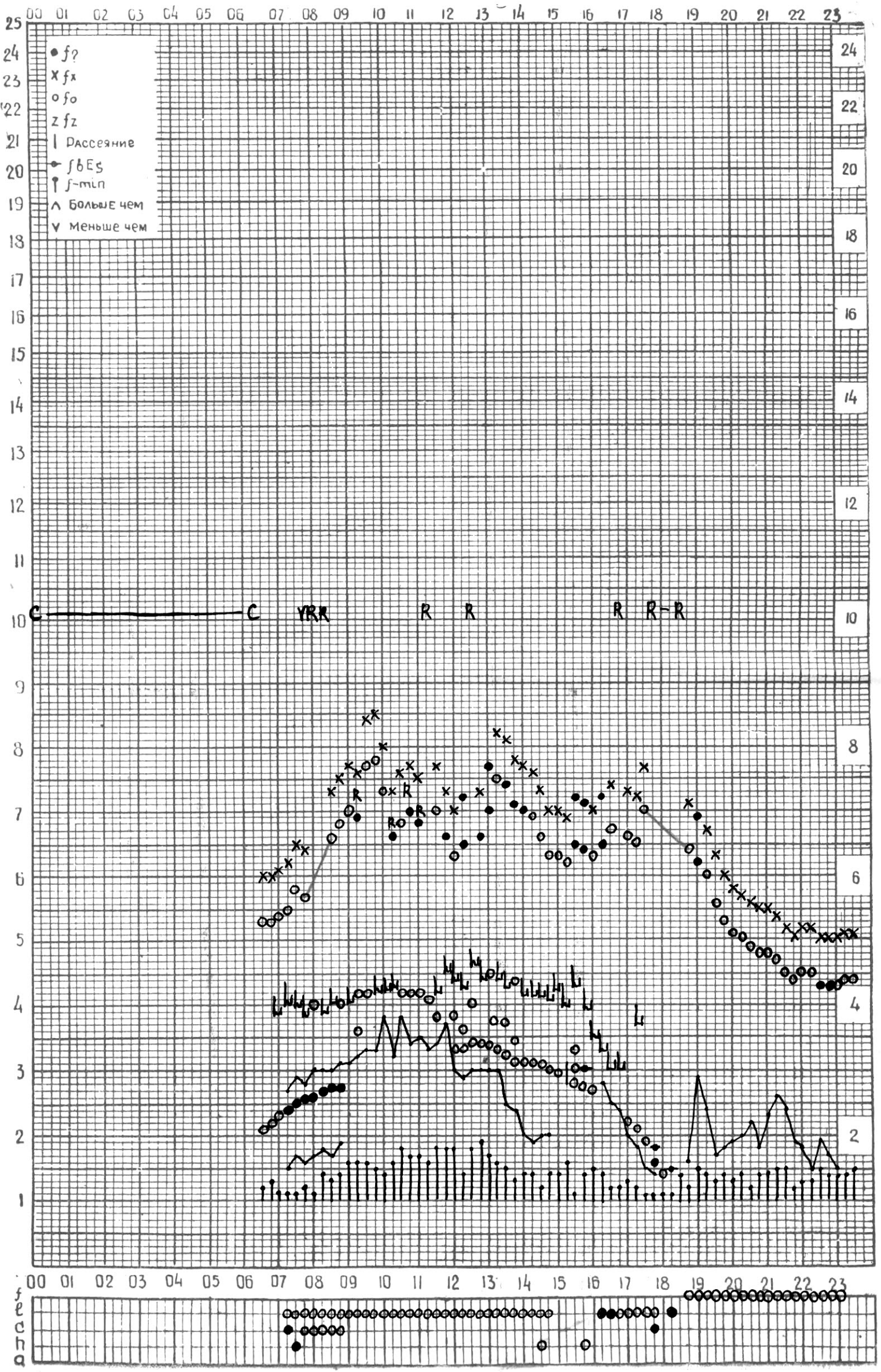
СТАНЦИЯ ТБИЛИСИ F-ГРАФИК ИОНОСФЕРНЫХ ДАННЫХ, ДАТА 20 СЕНТЯБРЯ 1973Г
