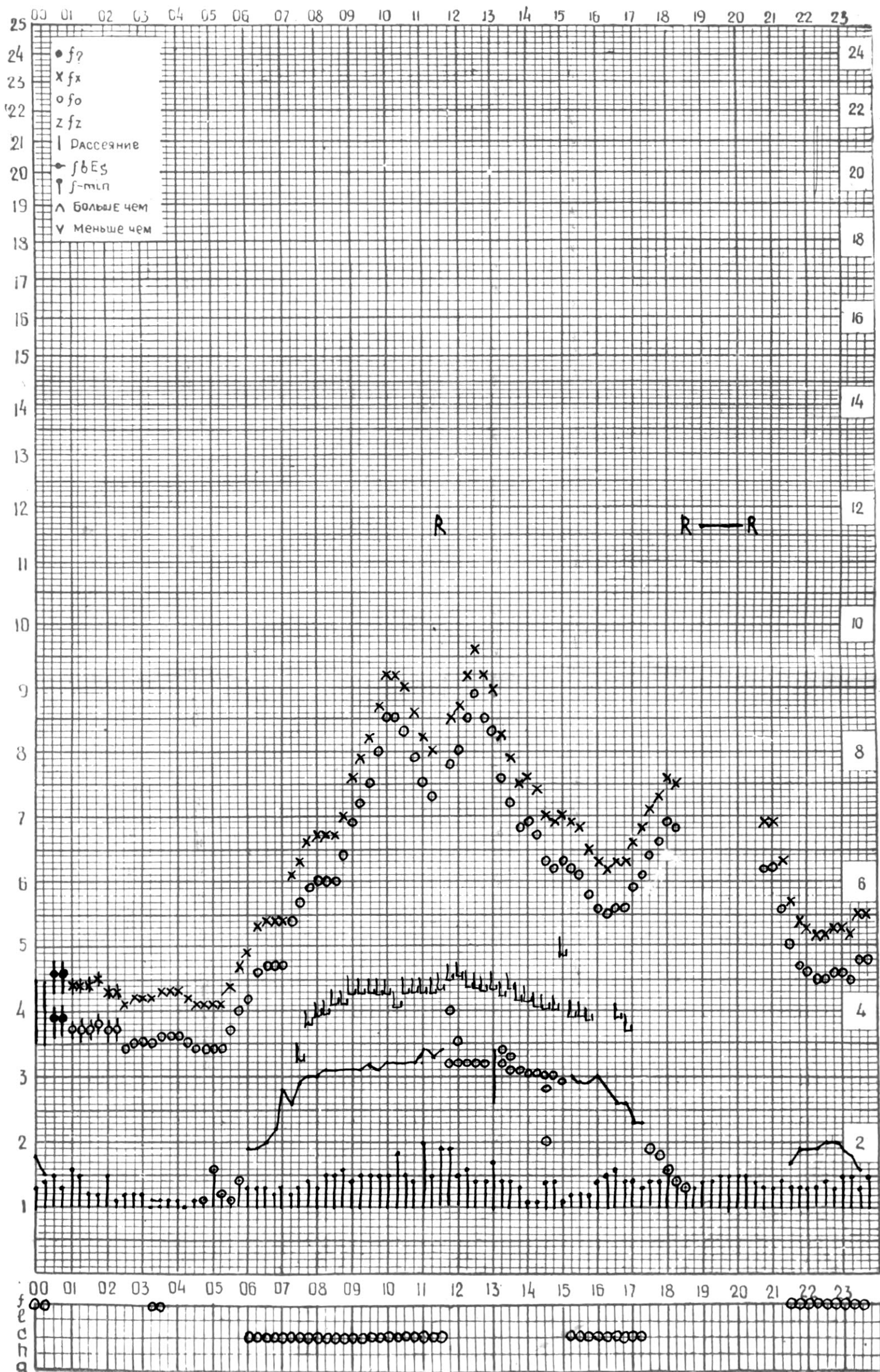
СТАНЦИЯ ТБИЛИСИ F—ГРАФИК ИОНОСФЕРНЫХ ДАННЫХ, ДАТА 17 СЕНТЯБРЯ 1973 Г
