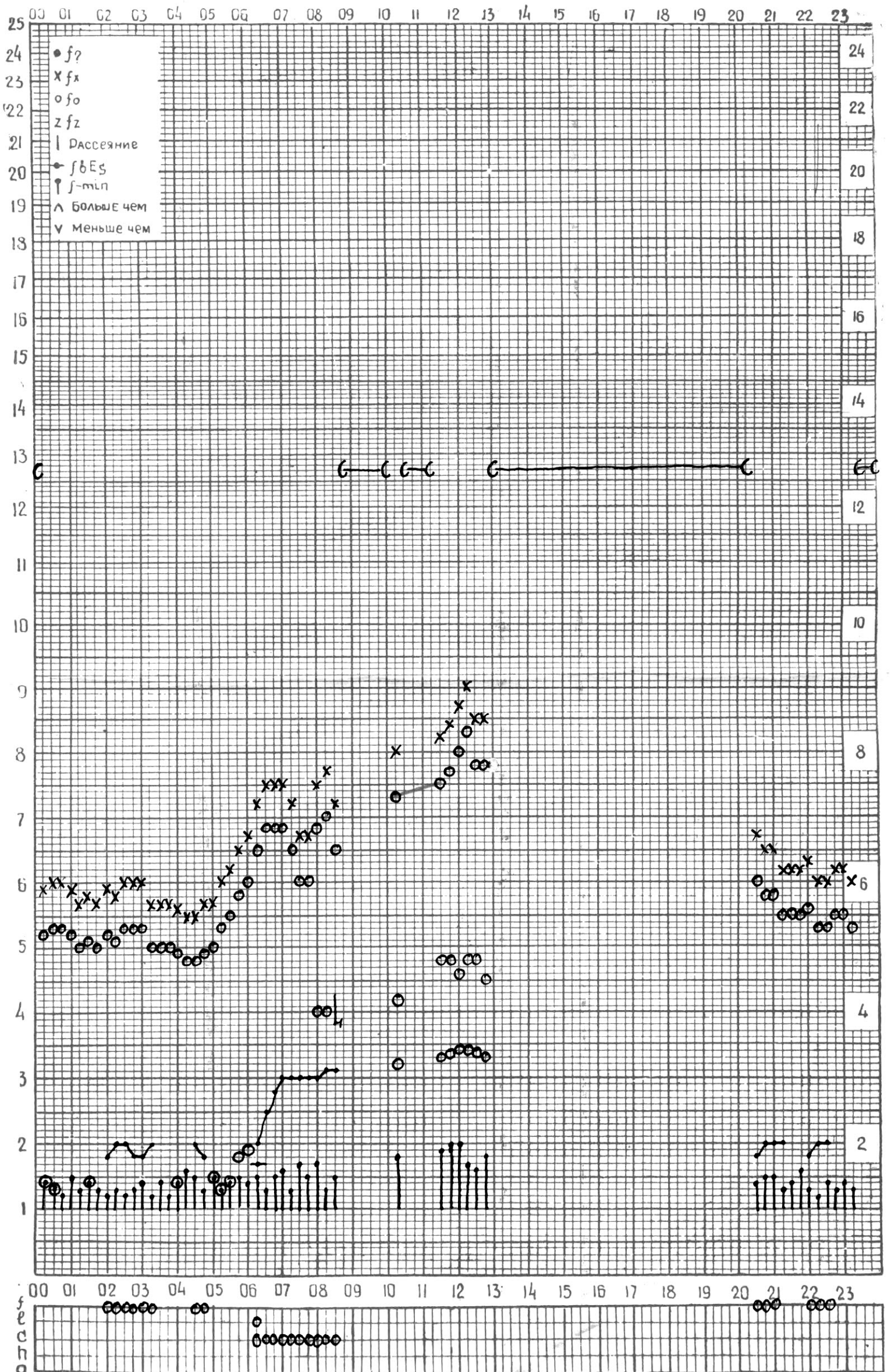
СТАНЦИЯ ТБИЛИСИ F-ГРАФИК ИОНОСФЕРНЫХ ДАННЫХ, ДАТА 8 СЕНТЯБРЯ 1973г
