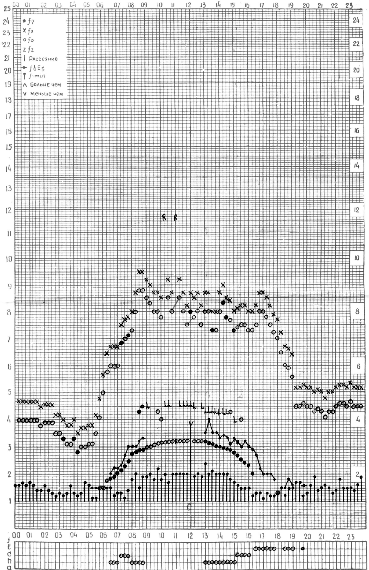
СТАНЦИЯ ТБИЛИСИ F—ГРАФИК ИОНОСФЕРНЫХ ДАННЫХ, ДАТА 27 СЕНТЯБРЯ 1973 Г
