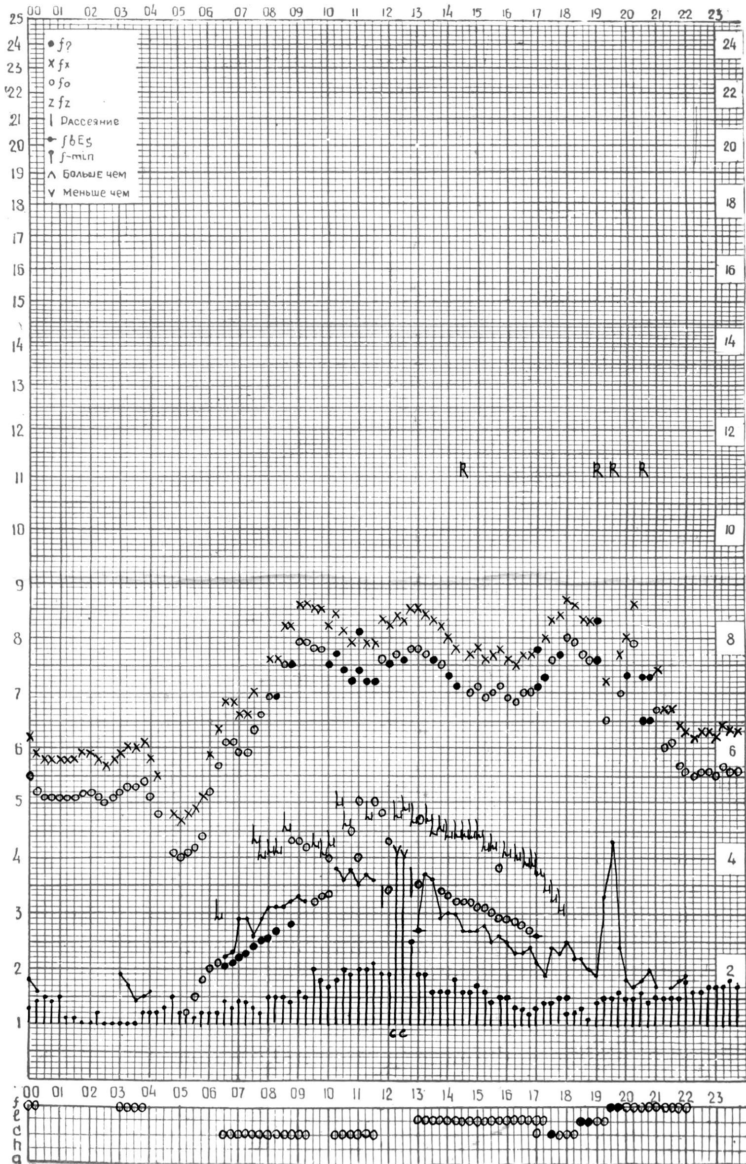
СТАНЦИЯ ТБИЛИСИ F-ГРАФИК ИОНОСФЕРНЫХ ДАННЫХ, ДАТА 6 СЕНТЯБРЯ 1973 Г
