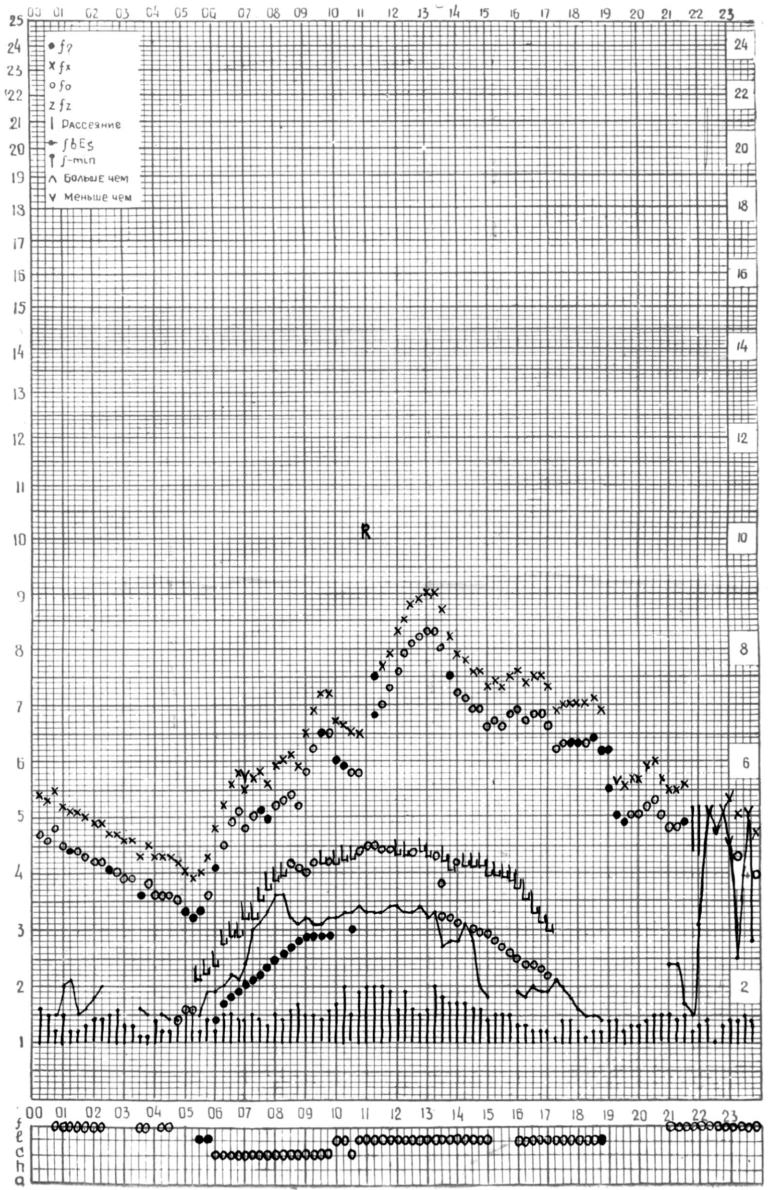
СТАНЦИЯ ТБИЛИСИ F-ГРАФИК ИОНОСФЕРНЫХ ДАННЫХ, ДАТА 16 СЕНТЯБРЯ 1973Г
