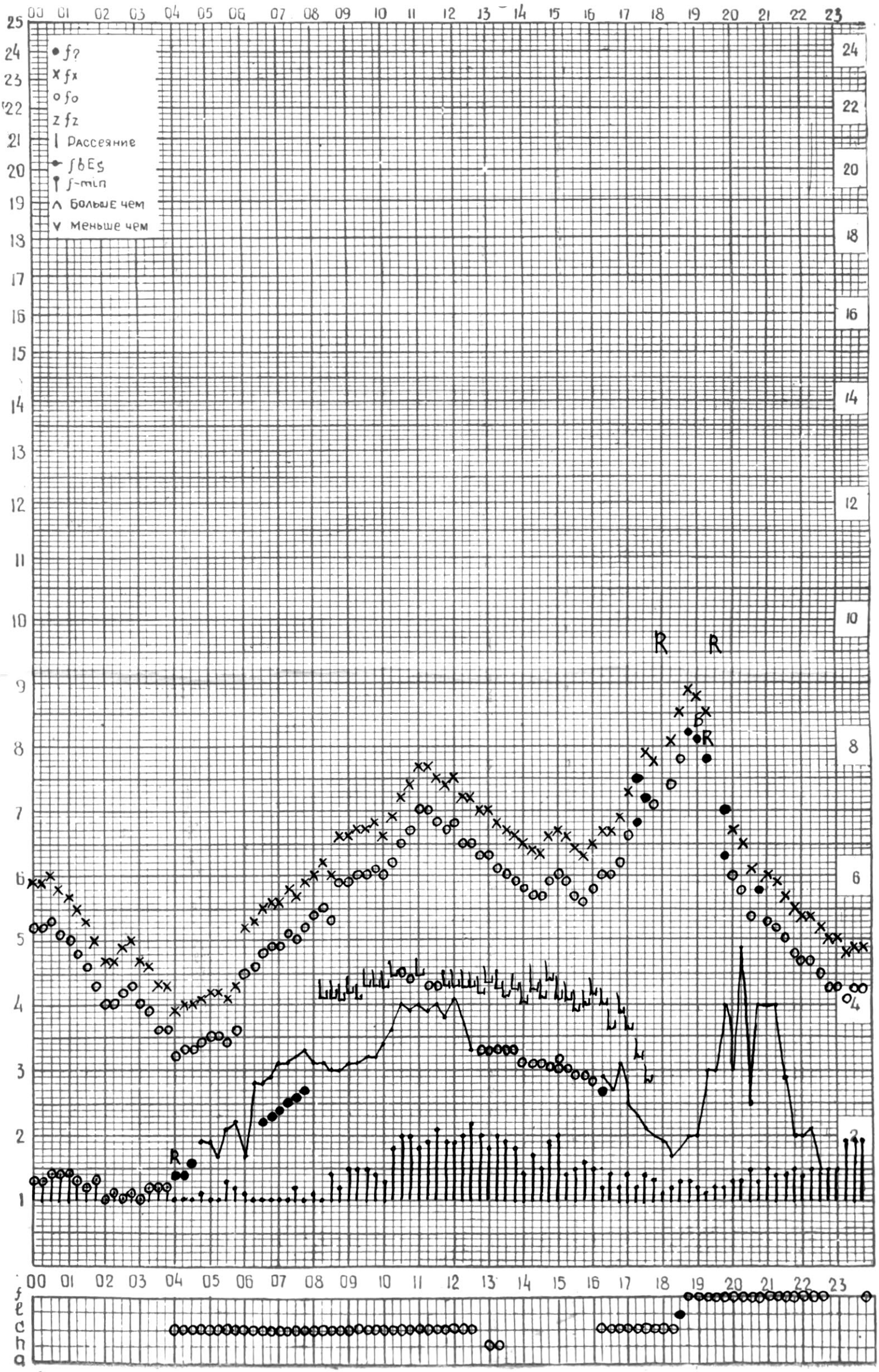
СТАНЦИЯ ТБИЛИСИ F-ГРАФИК ИОНОСФЕРНЫХ ДАННЫХ, ДАТА 10 СЕНТЯБРЯ 1973 Г
