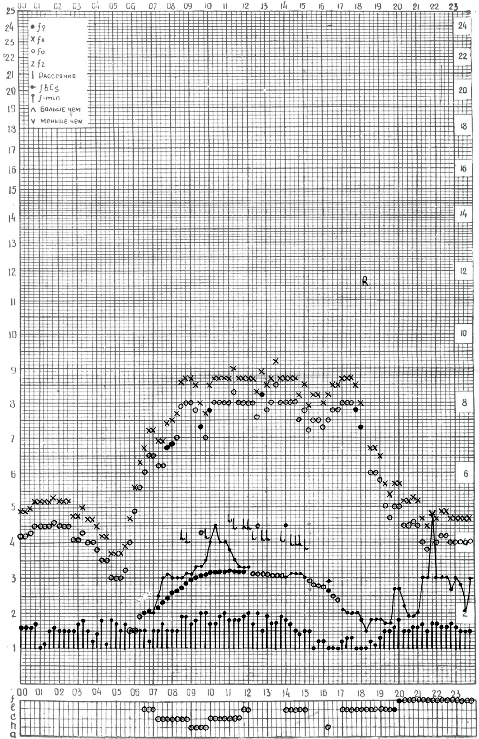
СТАНЦИЯ ТБИЛИСИ F-ГРАФИК ИОНОСФЕРНЫХ ДАННЫХ, ДАТА 24 СЕНТЯБРЯ 1973 Г
