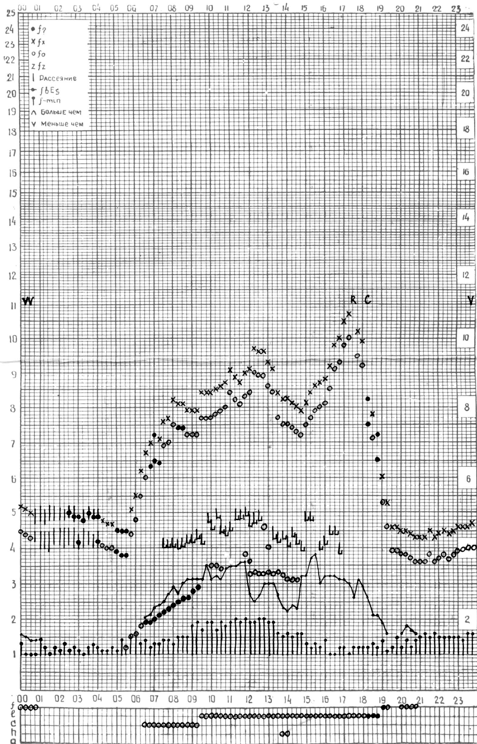
СТАНЦИЯ ТБИЛИСИ F-ГРАФИК ИОНОСФЕРНЫХ ДАННЫХ, ДАТА 28 СЕНТЯБРЯ 1973 Г
