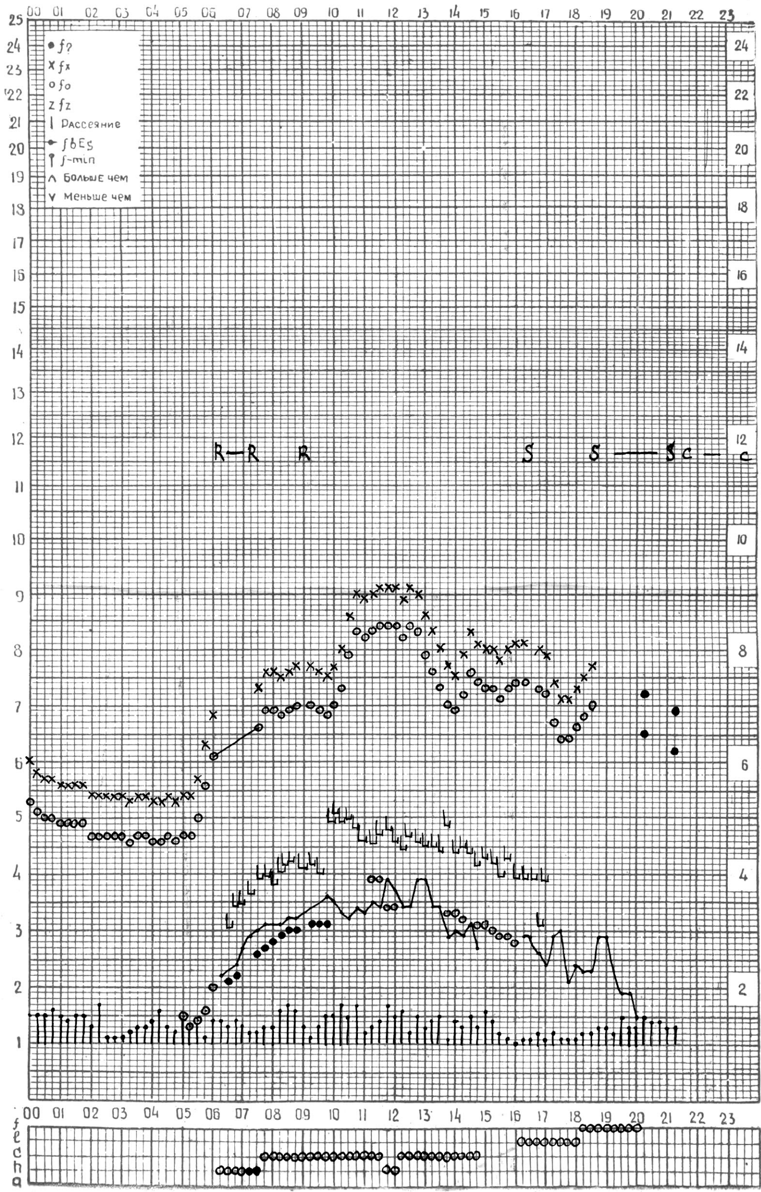
СТАНЦИЯ ТБИЛИСИ F-ГРАФИК ИОНОСФЕРНЫХ ДАННЫХ, ДАТА 9 СЕНТЯБРЯ 1973 Г
