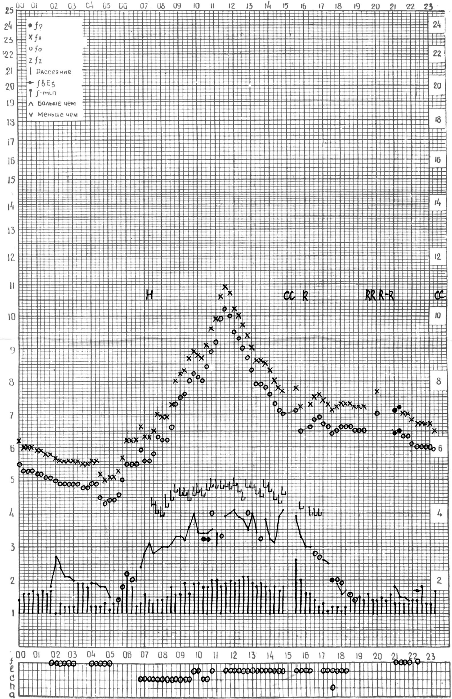
СТАНЦИЯ ТБИЛИСИ F-ГРАФИК ИОНОСФЕРНЫХ ДАННЫХ, ДАТА 7 СЕНТЯБРЯ 1973 Г
