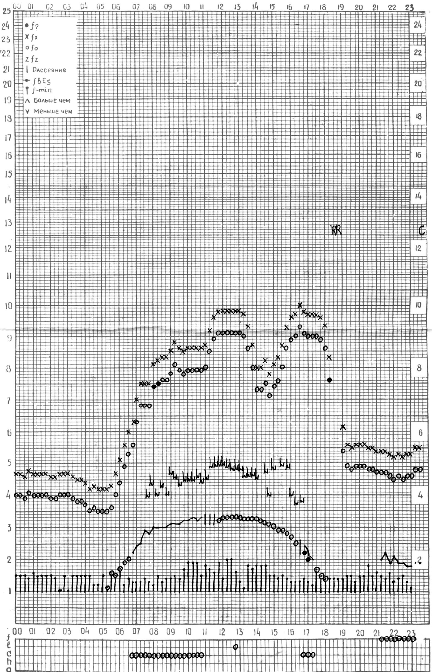
СТАНЦИЯ ТБИЛИСИ F-ГРАФИК ИОНОСФЕРНЫХ ДАННЫХ, ДАТА 29 СЕНТЯБРЯ 1973г
