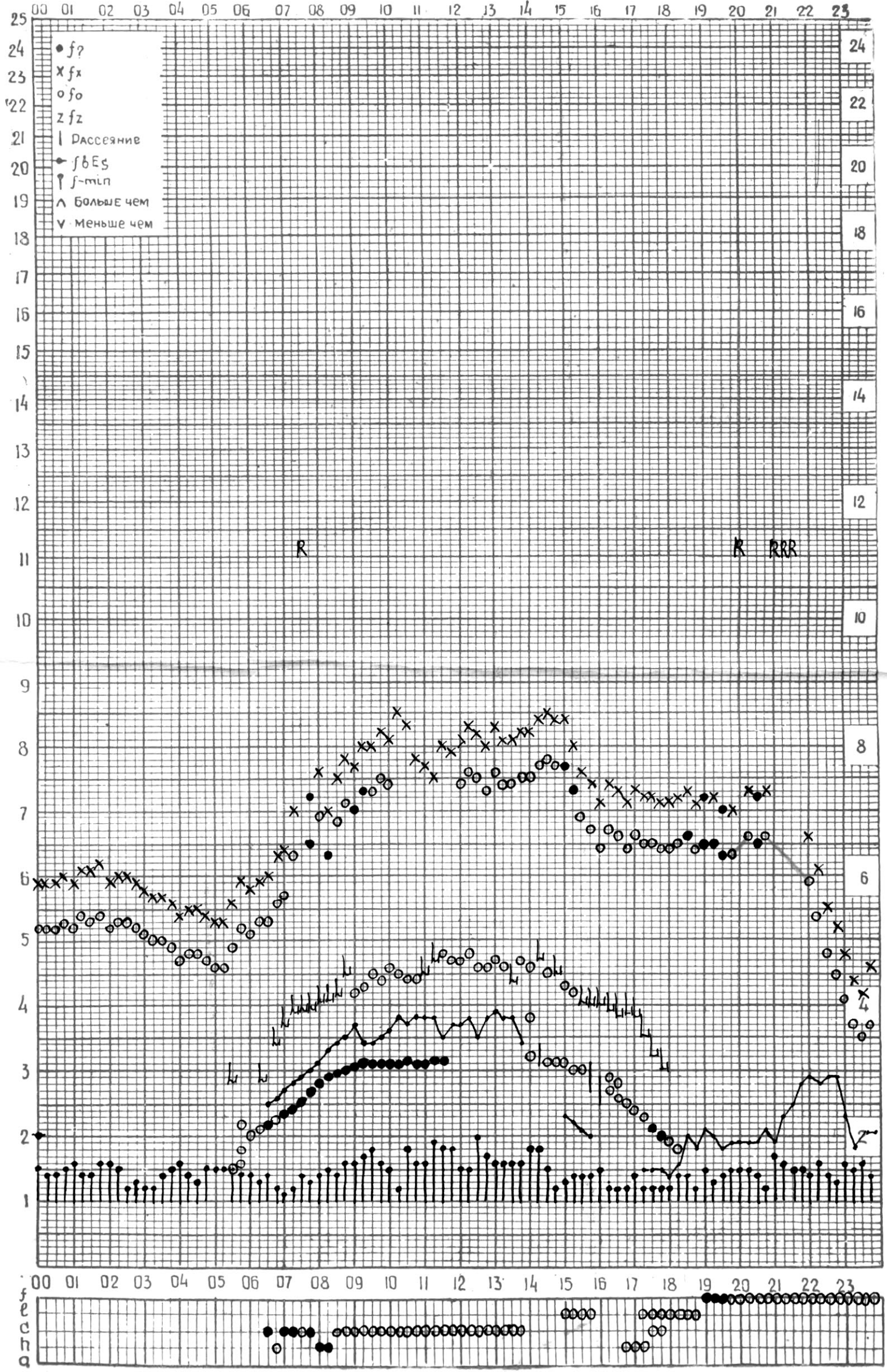
СТАНЦИЯ ТБИЛИСИ F-ГРАФИК ИОНОСФЕРНЫХ ДАННЫХ, ДАТА 1 СЕНТЯБРЯ 1973 Г
