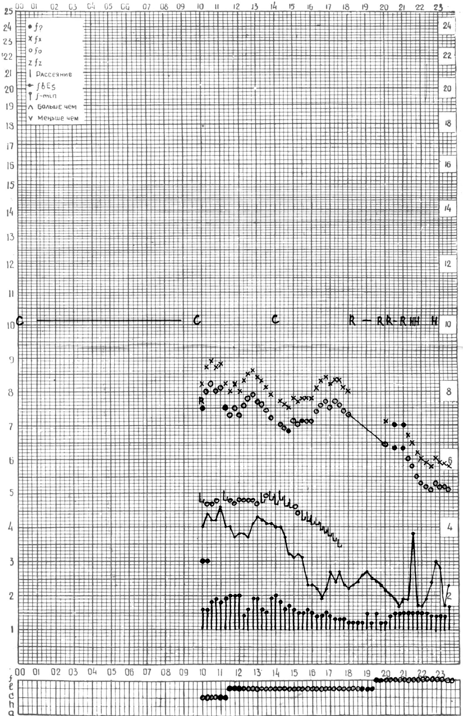
СТАНЦИЯ ТБИЛИСИ F-ГРАФИК ИОНОСФЕРНЫХ ДАННЫХ, ДАТА 3 СЕНТЯБРЯ 1973 Г
