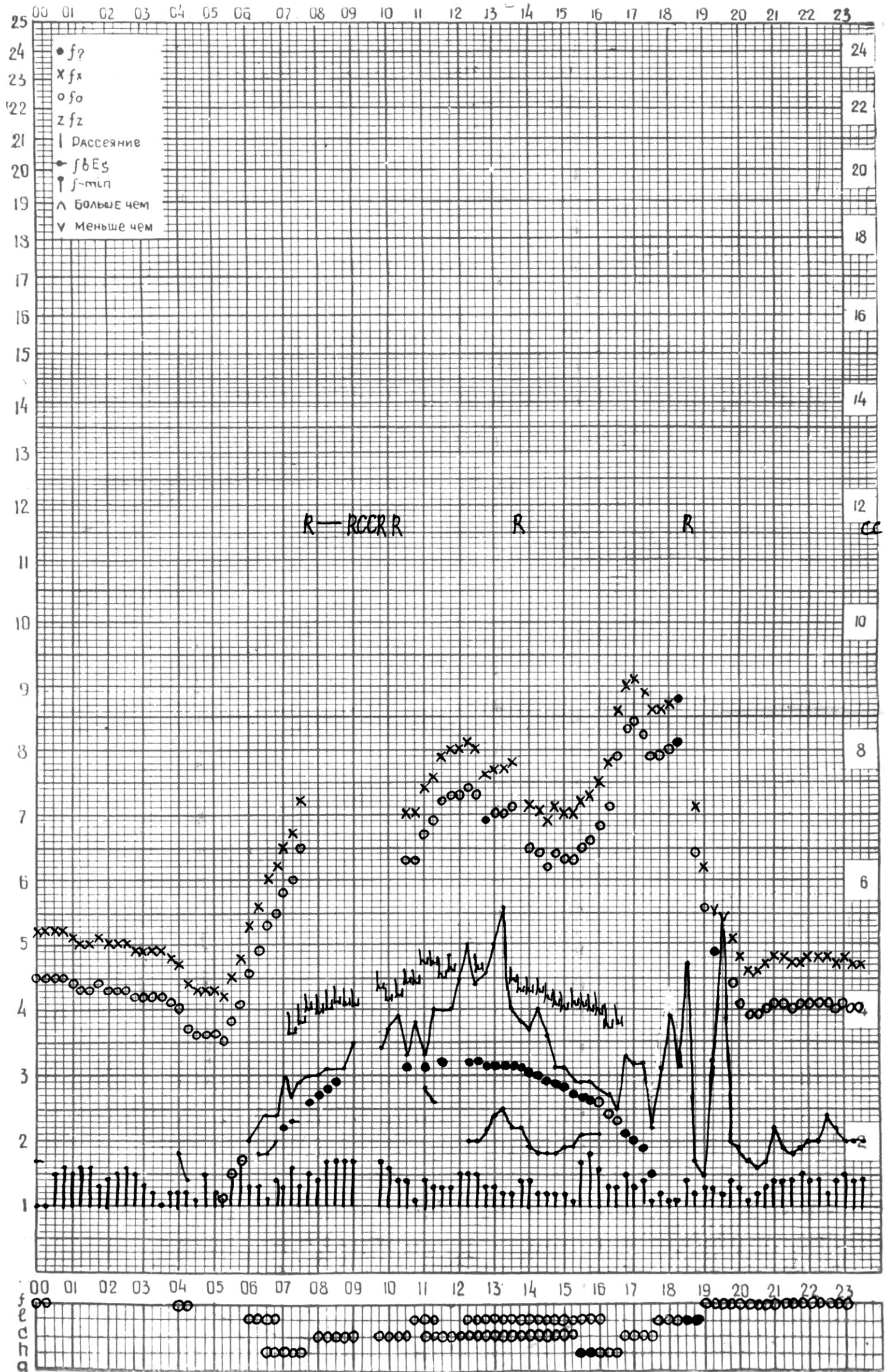
СТАНЦИЯ ТБИЛИСИ F-ГРАФИК ИОНОСФЕРНЫХ ДАННЫХ, ДАТА 21 СЕНТЯБРЯ 1973 Г
