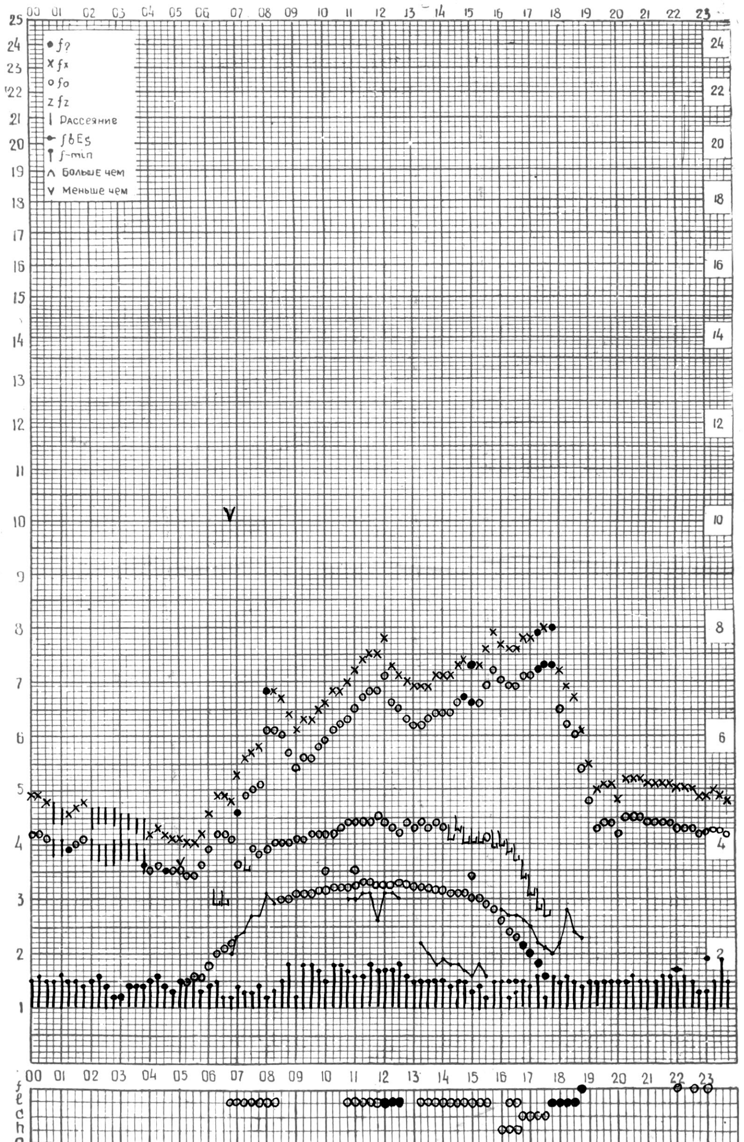
СТАНЦИЯ ТБИЛИСИ F-ГРАФИК ИОНОСФЕРНЫХ ДАННЫХ, ДАТА 14 СЕНТЯБРЯ 1973Г
