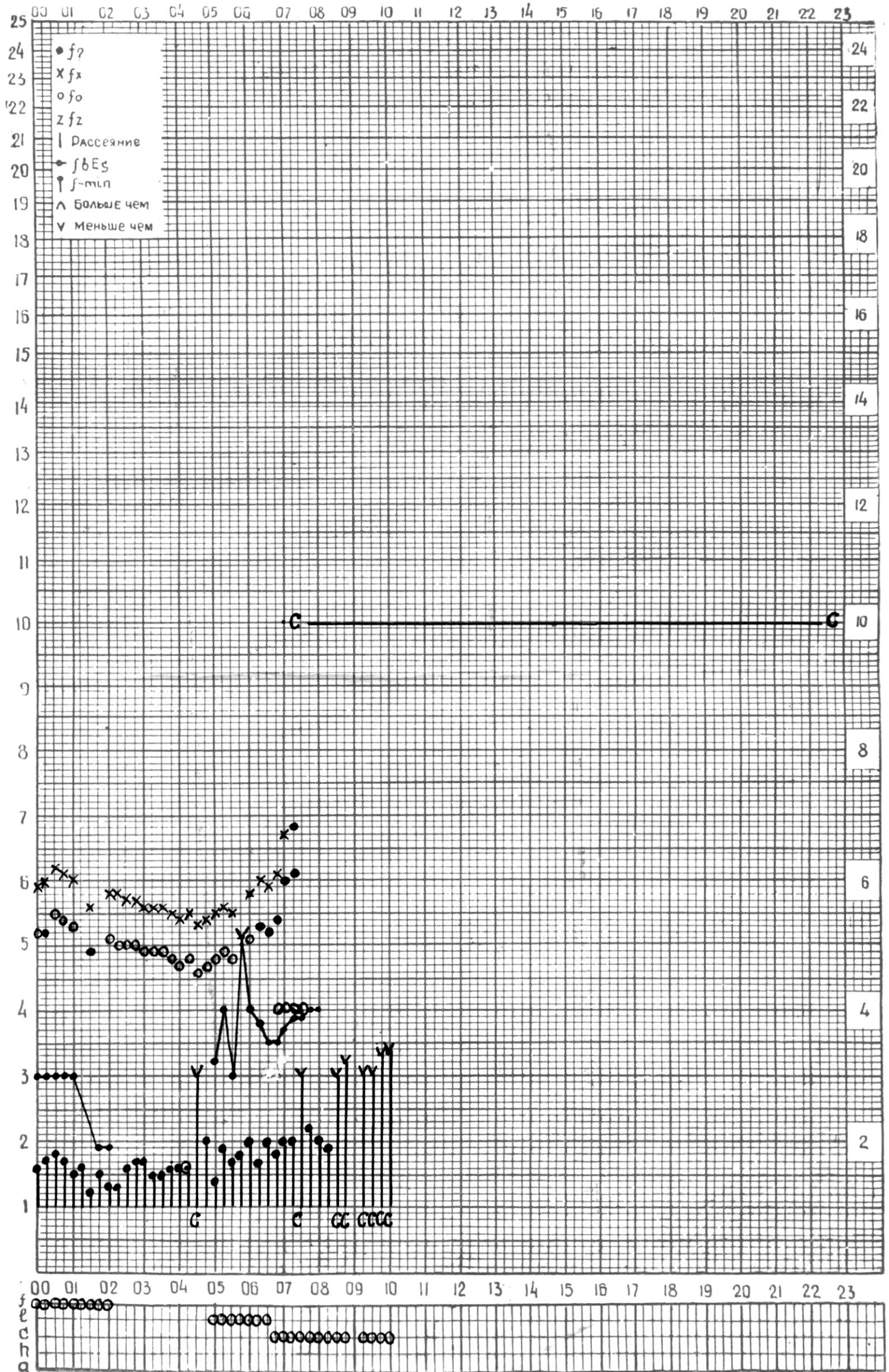
СТАНЦИЯ ТБИЛИСИ F-ГРАФИК ИОНОСФЕРНЫХ ДАННЫХ, ДАТА 8 ИЮЛЯ 1973Г
