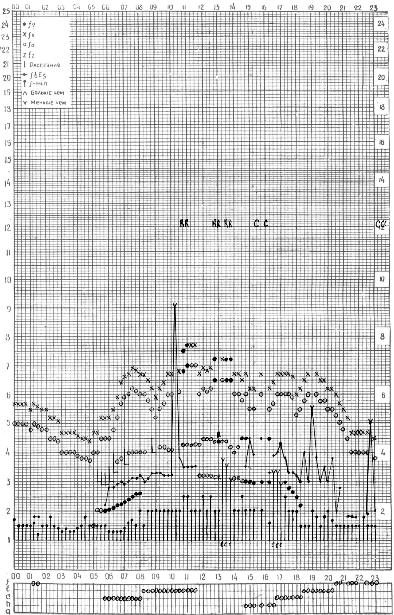
СТАНЦИЯ ТБИЛИСИ F-ГРАФИК ИОНОСФЕРНЫХ ДАННЫХ, ДАТА 29 ИЮЛЯ 1973 Г
