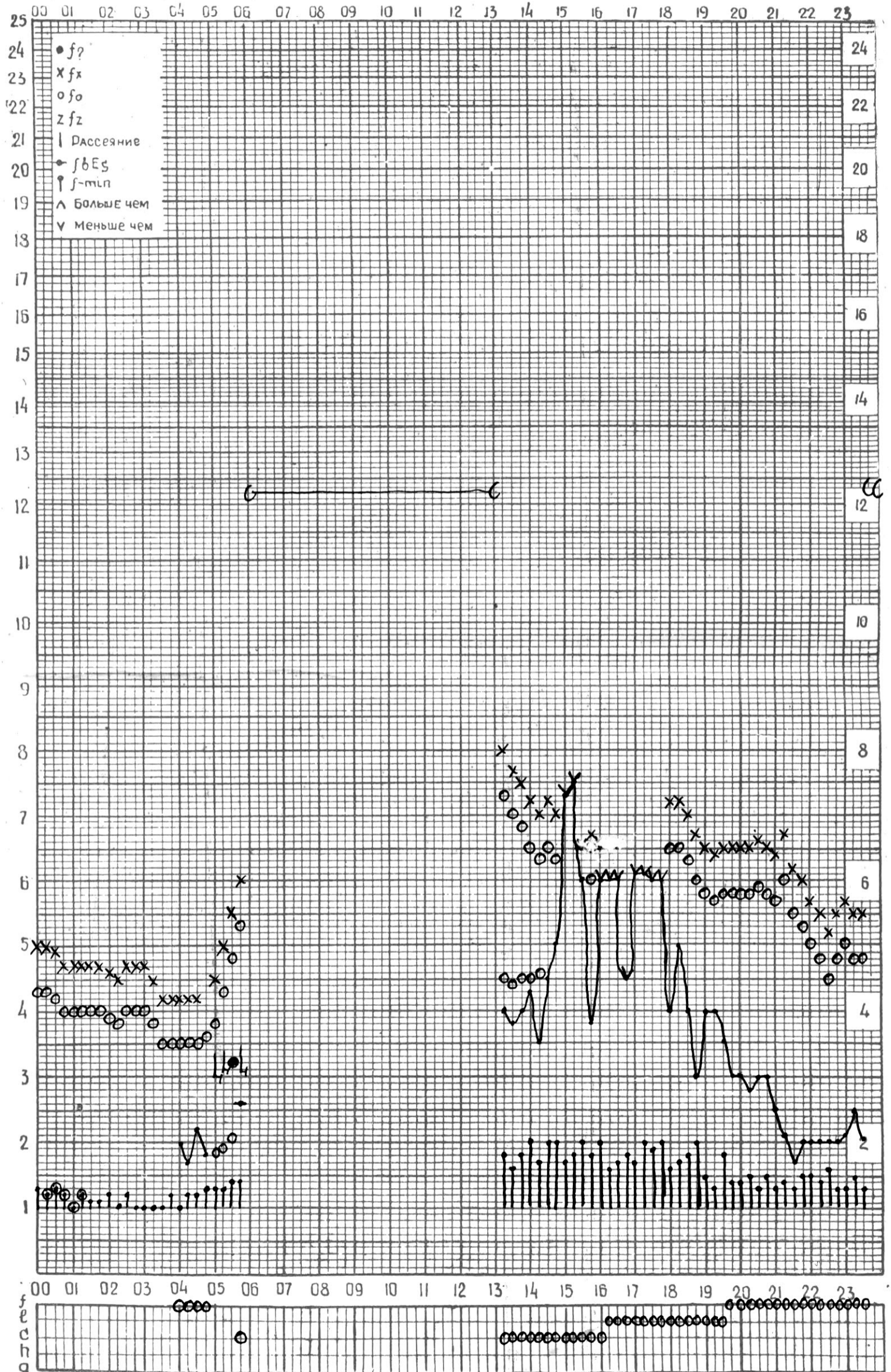
СТАНЦИЯ ТБИЛИСИ F-ГРАФИК ИОНОСФЕРНЫХ ДАННЫХ, ДАТА 18 ИЮЛЯ 1973Г
