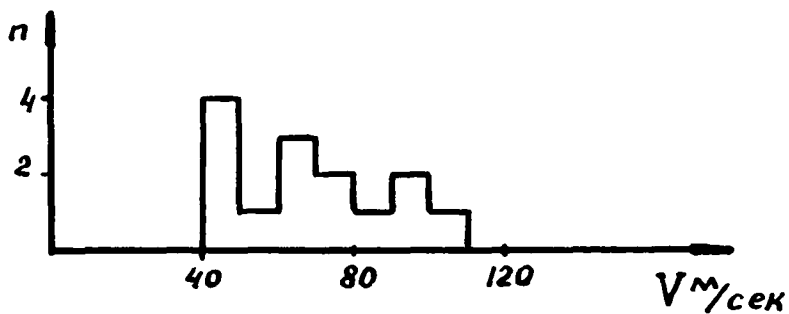
Гистограмма распределения величин скоростей дрейфа ионосферных неоднородностей за февраль 1961 года слой E, ст. Ашхабад.
