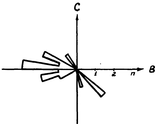
„Роза ветров“ за февраль 1961 г. слой E, ст. „Ашхабад“
